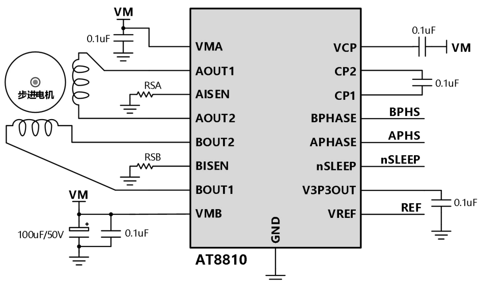
有检流电阻应用
