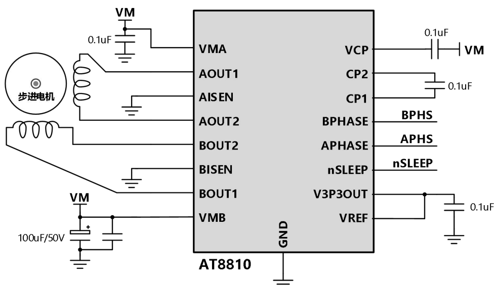
无检流电阻应用
